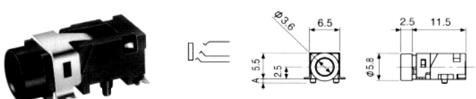
No.M03-663A0 (3.5φ) STEREO
