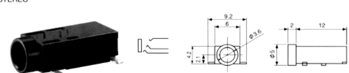
No.M03-836F0 (3.5φ) STEREO
