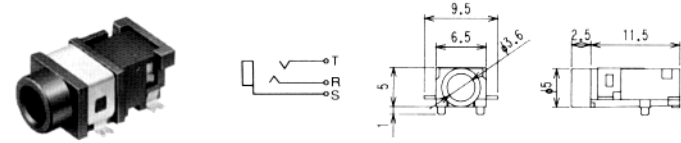
No.M03-772A0 (3.5φ) STEREO
