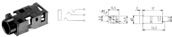
No.M03-772A0 (3.5φ) STEREO
